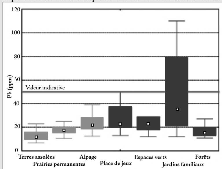
Figure 2: Comparaison des teneurs en plomb entre différentes utilisations du sol
